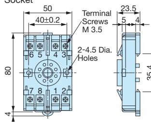
Socket
